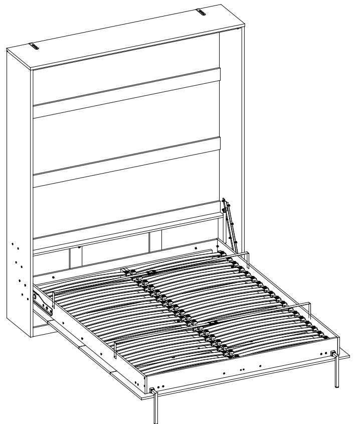
0203 140V 160,7x223,5x224,5 cm
